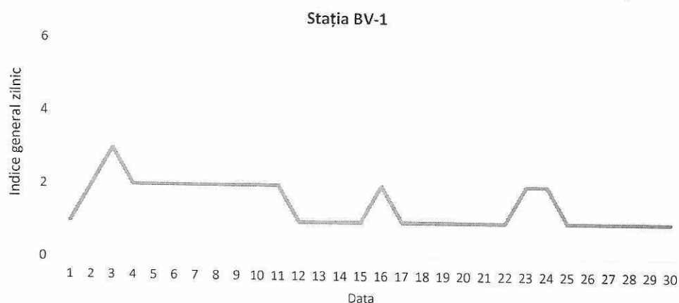
Figura 13. Evoluția indicelui general de calitate aerului din stația BV-1
