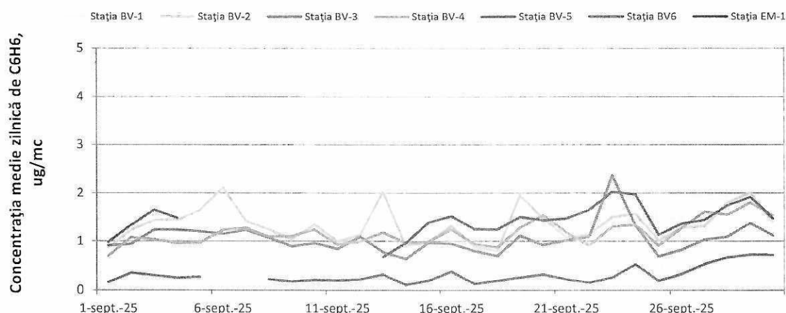
Figura 7. Evoluția concentrațiilor medii zilnice de benzen în luna septembrie 2025
