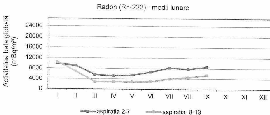
Figura 22. Activitatea calculată a Radonului
