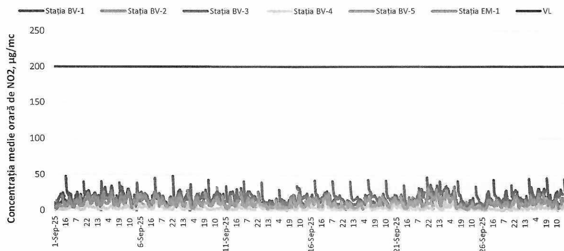
Figura 3. Concentrații medii orare de NO 2 în luna septembrie 2025
