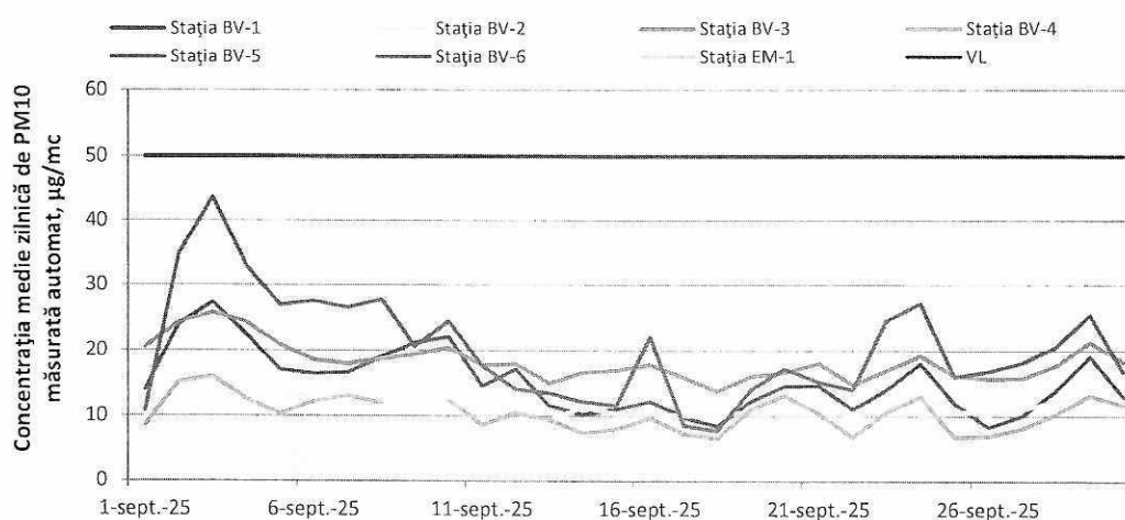
Figura 10. Evoluția concentrațiilor medii zilnice de PM 10 automat în luna septembrie 2025
