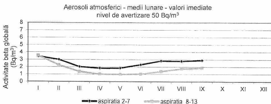
Figura 21. Activitatea beta globală pentru aerosoli atmosferici
