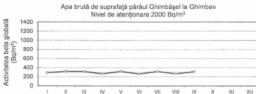
Figura 25. Activitatea beta globală imediată pentru apa de suprafață Pârâul Ghimbășel
