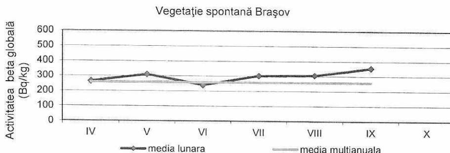
Fig. 29. Activitatea beta globală la 5 zile pentru vegetația spontană
