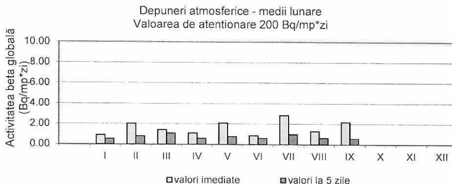
Figura 24. Activitatea beta globală pentru depuneri atmosferice
