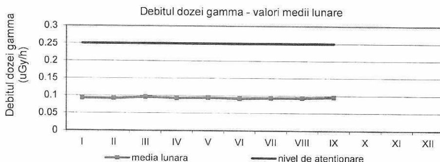
Figura 23. Debitul dozei gamma
