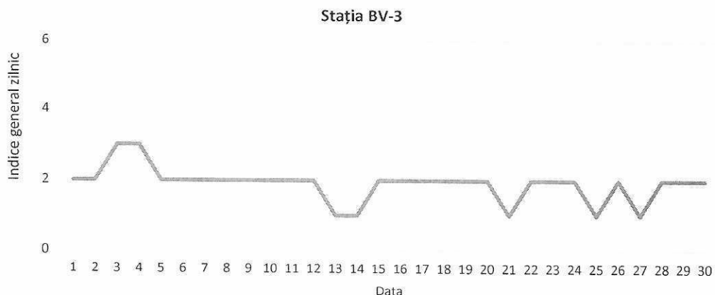
Figura 15. Evoluția indicelui general de calitate aerului din stația BV-3
