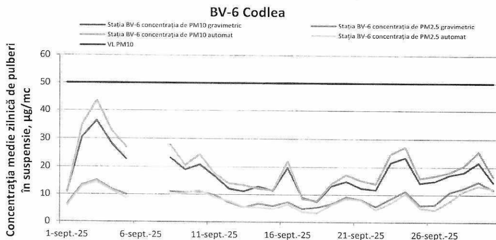
Figura 12. Evoluția concentrațiilor medii zilnice de PM 10 gravimetric și automat și PM 2,5 gravimetric și automat în stația de fond urban BV-6 în luna septembrie 2025
