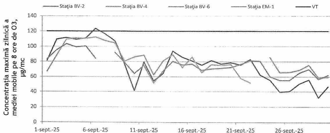
Figura 5. Evoluția concentrațiilor maximelor zilnice ale mediilor mobile pe 8 ore de O 3 în luna septembrie 2025
