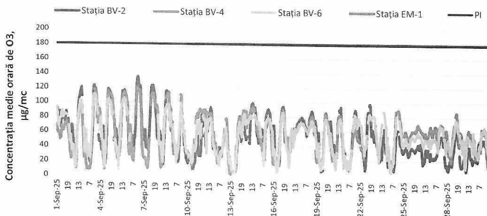
Figura 6. Evoluția concentrațiilor medii orare de O 3 în luna septembrie 2025
