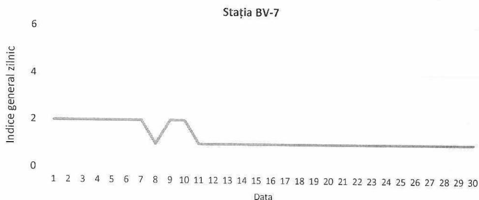
Figura 19. Evoluția indicelui general de calitate aerului din stația BV-7
