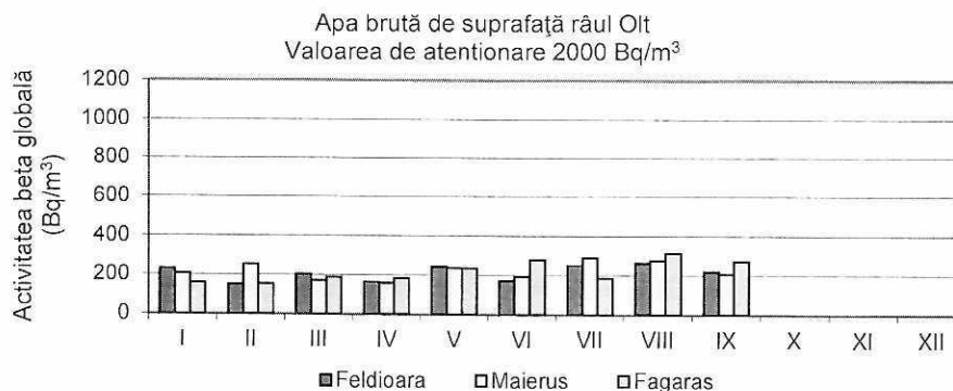
Fig. 27. Activitatea beta globală la 5 zile pentru apa de suprafață Râul Olt
