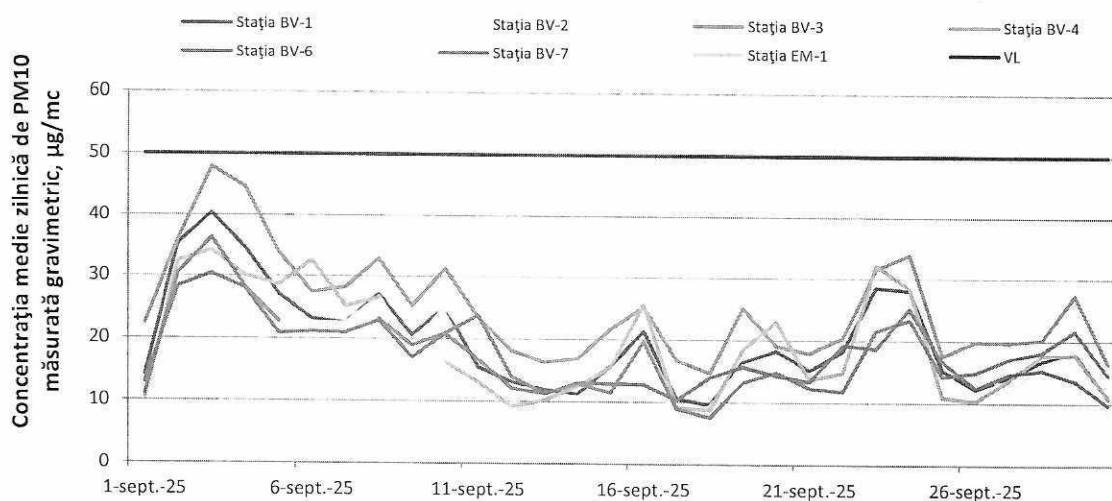
Figura 8. Evoluția concentrațiilor medii zilnice de PM10 (gravimetric) în luna septembrie 2025
