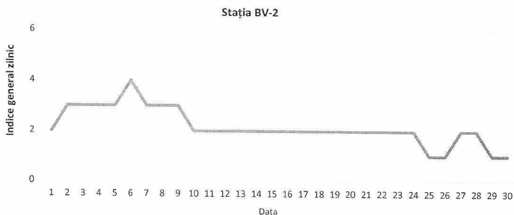
Figura 14. Evoluția indicelui general de calitate aerului din stația BV-2
