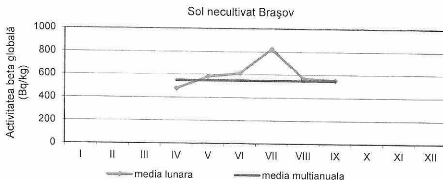
Fig. 28. Activitatea beta globală la 5 zile pentru solul necultivat
