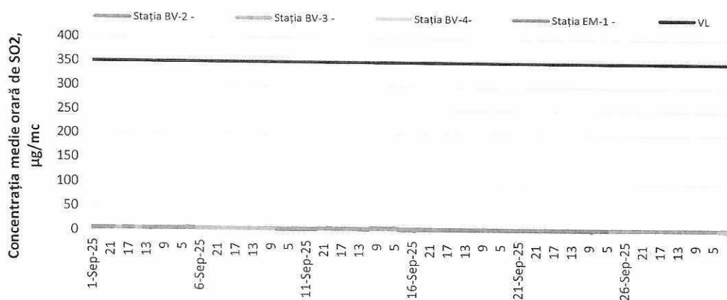
Figura 2. Evoluția mediilor orare de SO 2 în luna septembrie 2025
